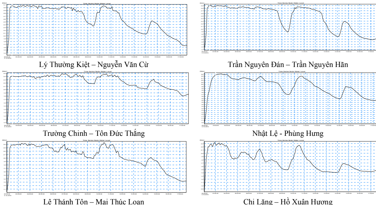
Hình 9. Đường quá trình mực nước một số tuyến đường đô thị Huế
