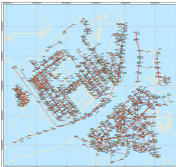
Hình 2. Bản đồ hệ thống thoát nước
