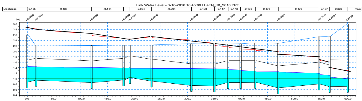
Hình 8. Độ sâu ngập lớn nhất trên các tuyến đường đô thị Huế
